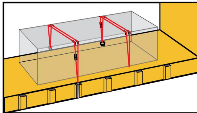
MÉTHODE DE DOUBLE ARRIMAGE DESSIN 5
