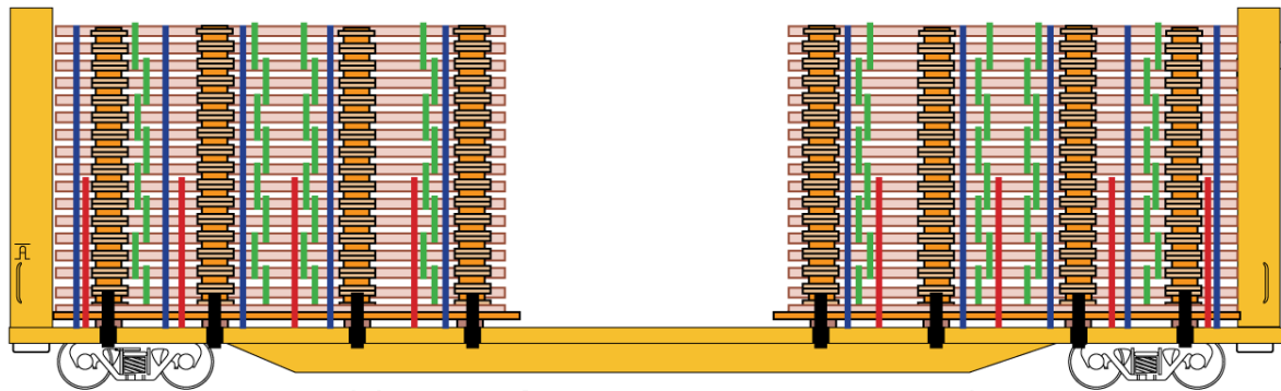
DESSIN 1: CHARGEMENT: 2 PILES
