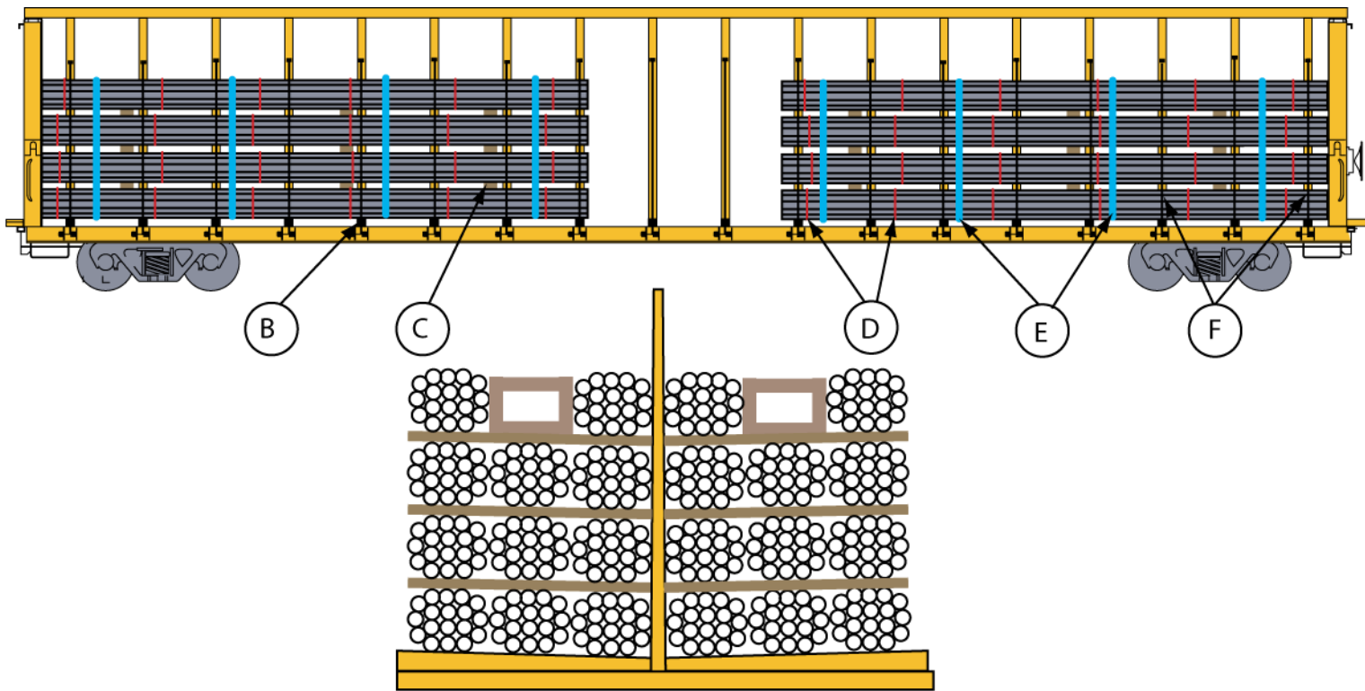
DESSIN 1 (ARRIMAGE NON MONTRE)
